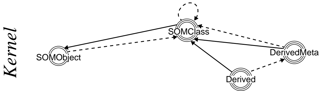
Figure 7. Additional SOM kernel metaclasses required for SOM derived metaclasses.
